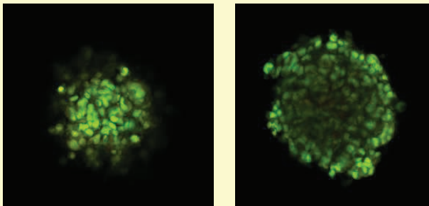
Konfokale Fluoreszenzaufnahmen eines Tumorzell-Sphäroids in unterschiedlicher Probentiefe (Hochschule Aalen)
